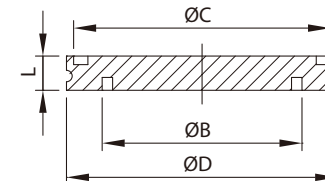
ISO-Blank Flange
